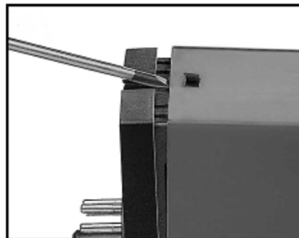
Рис. 1: Отделение задней панели от корпуса
